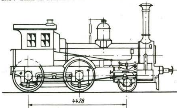
Bild 4 Skizze der Lokomotiven der BAE-Nr. 85—88
