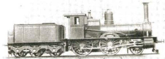
Bild 10 Ansicht einer Lokomotive aus der Lieferserie Nr. 118—122 Skizzen: Hans Köhler, Erfurt Fotos: Repros Werkaufnahmen
