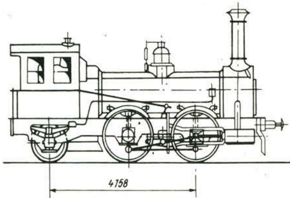
Bild 2 Desgleichen für die Lieferung der Nr. 89—96 und 108—117 (?)
